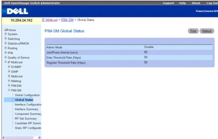
그림 12-34. PIM-SM 전역 상태
