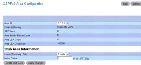
그림 10-19. OSPFv3 스태 영역 구성
