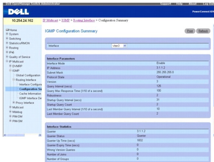
그림 12-9. 라우팅 구성 요약
