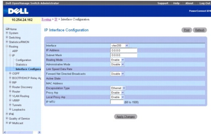
그림 9-5. IP 인터페이스 구성
