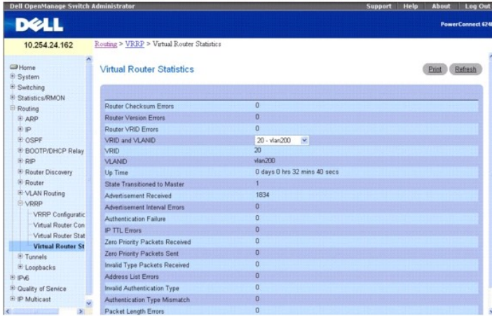
그림 9-41. 가상 라우터 통계
