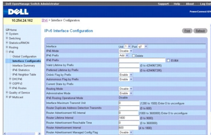
그림 10-2. IPv6 인터페이스 구성
